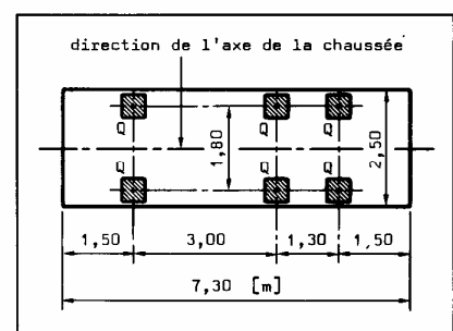
Fig. 2. — Géométrie du modèle de charge 1.
